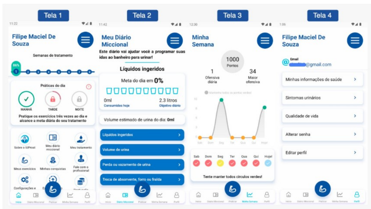
Figura 3.5: Telas principais do IUProst: Versão 2.0.
